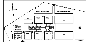
Übersichtsplan Messegebäude
